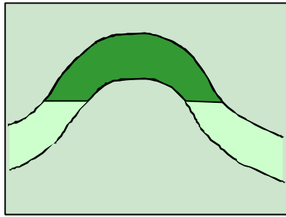
A. Anticline, dome
